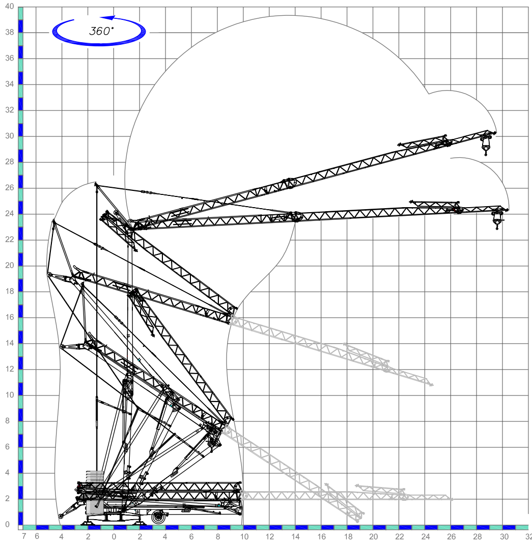
Sequenza di montaggio su 360°. Aufstellvorgang über 360°. Dérèlement de montage sur 360°. Erection procedure on 360°. Montaje sobre 360°.
